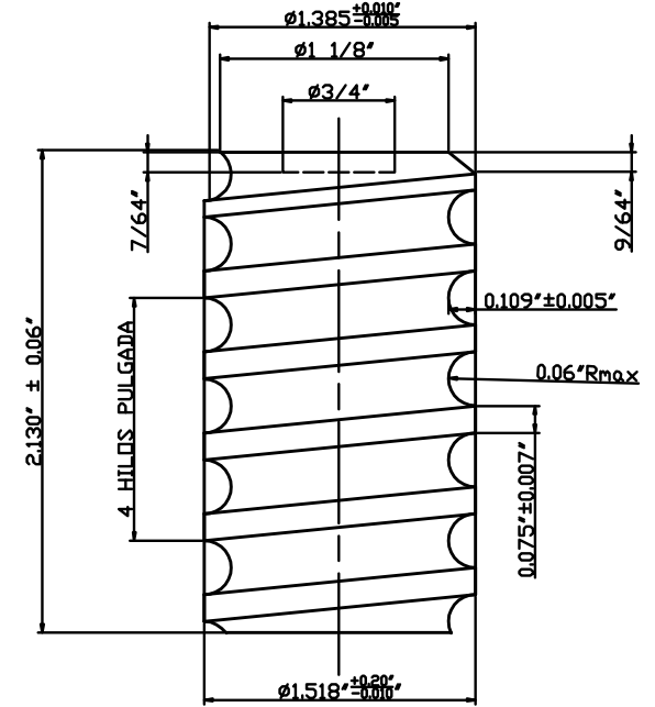
CAPSULA Ø1 3/8" (VER NOTA 3) DETALLE B
