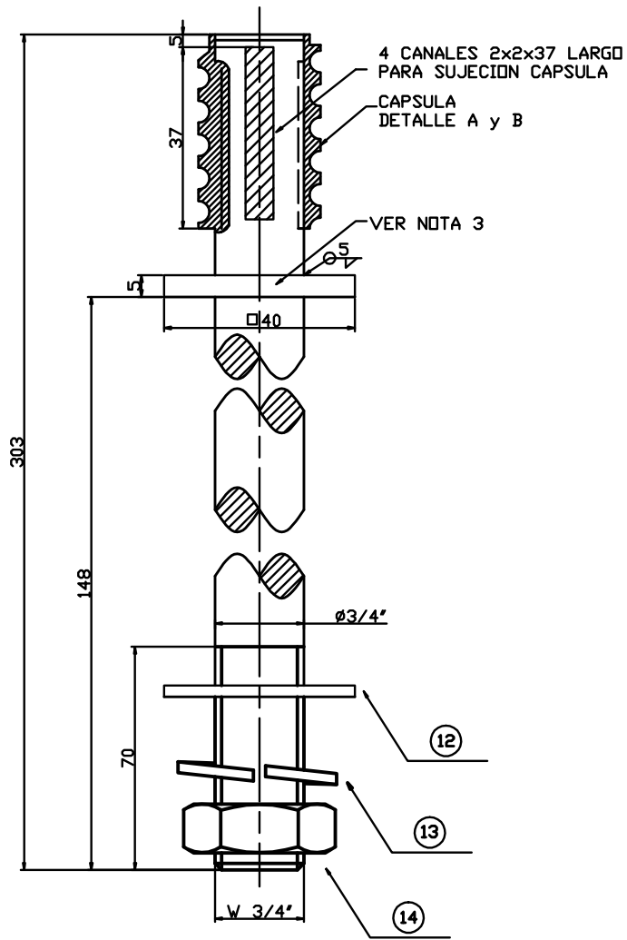
CAPSULA Ø1" (VER NOTA 3) DETALLE A
