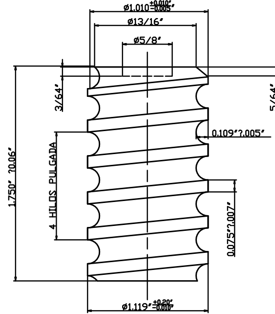
CAPSULA Ø1" (VER NOTA 3) DETALLE A
