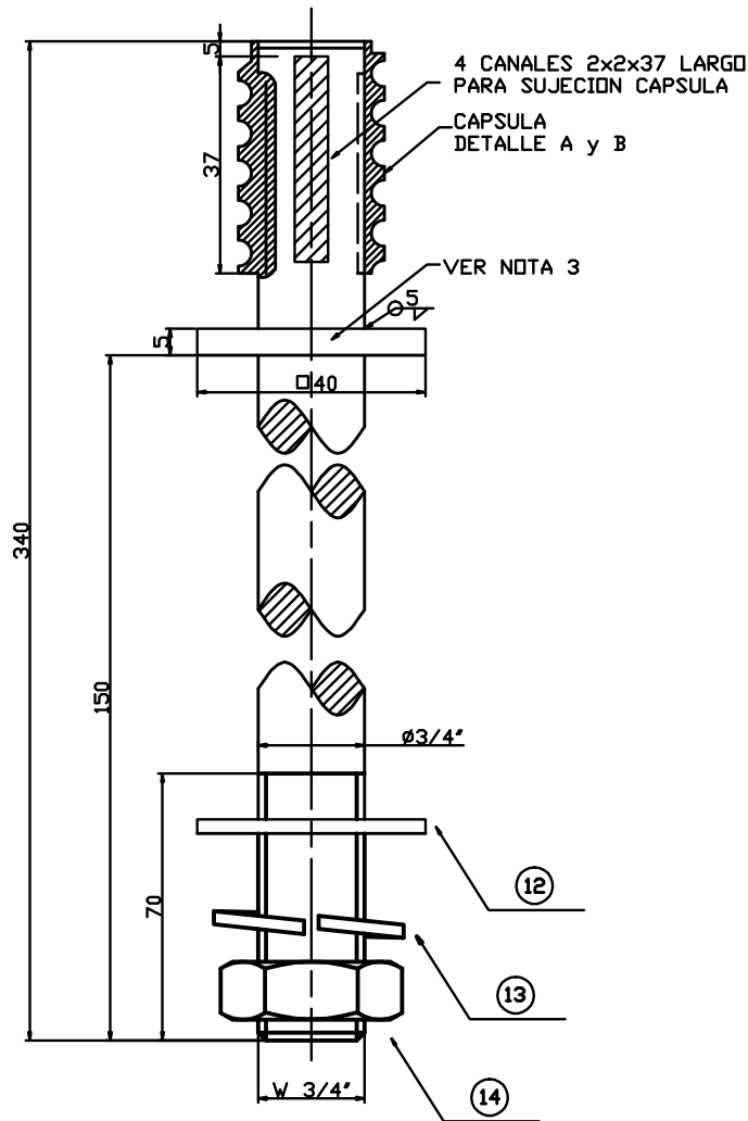
CAPSULA \phi 1" (VER NOTA 3) DETALLE A
