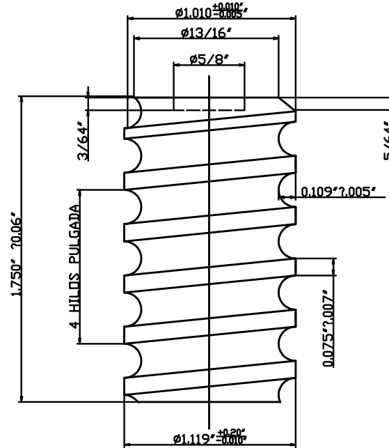
CAPSULA \phi 1" (VER NOTA 3) DETALLE A
