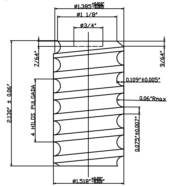
CAPSULA \phi 1 3/8" (VER NOTA 3) DETALLE B
