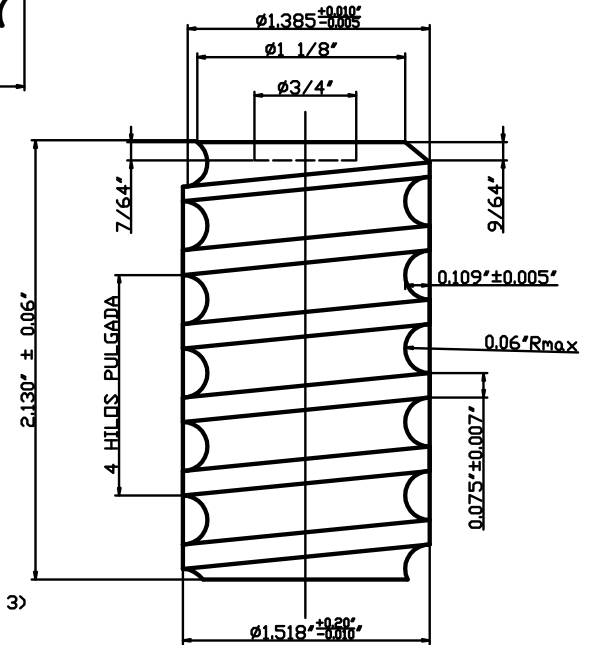
CAPSULA Ø1" (VER NOTA 3) DETALLE A
