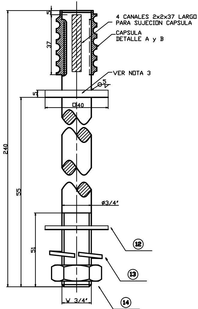
CAPSULA Ø1" (VER NOTA 3) DETALLE A
